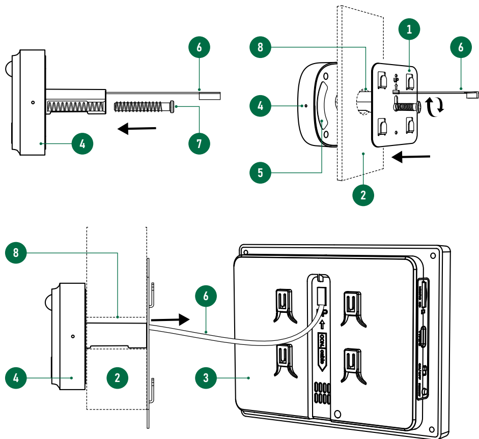
Рис.3 Установка видеоглазка
