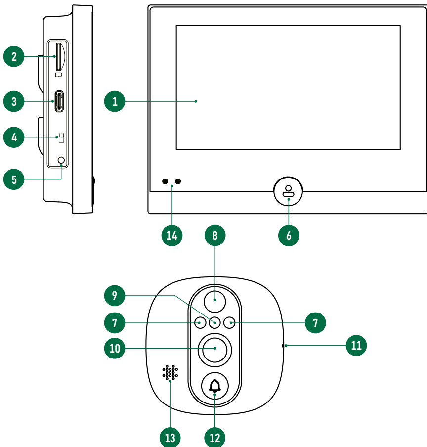
Рис.2 Описание видеоглазка FOCUS 4 WIFI KIT LITE
